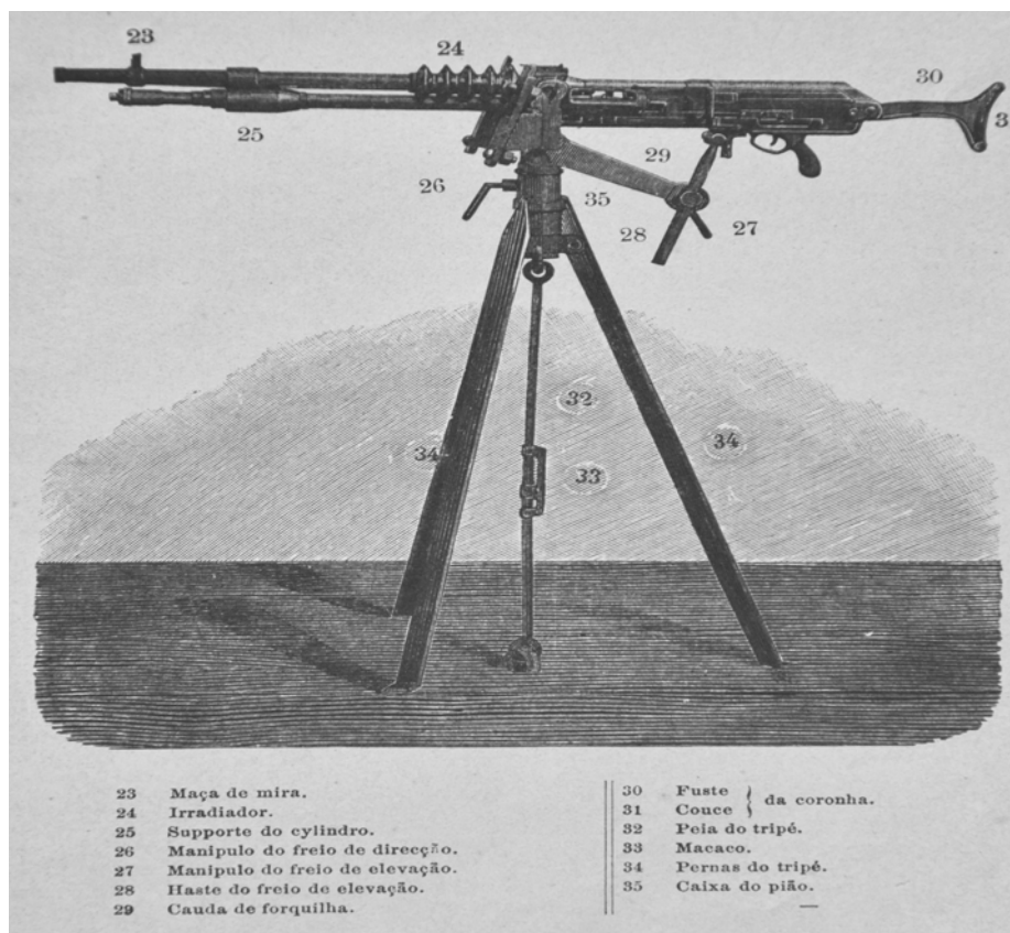
Fig. 12 - Gravura com representação da metralhadora Hotchkiss calibre 6,5 mm utilizada pela Armada, montada em reparo naval.
